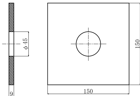
6. メッキ付角座金 (溶融亜鉛めっき HDZ 55)
