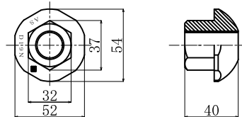
2. ASメッキコマナット D19N (溶融亜鉛めっき HDZ 35)
