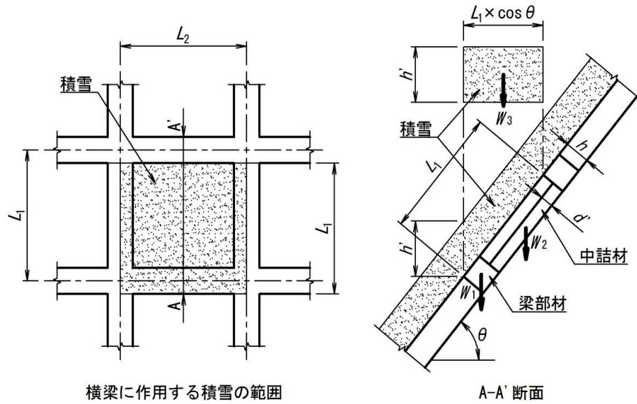
図1-2 積雪荷重の考え方
